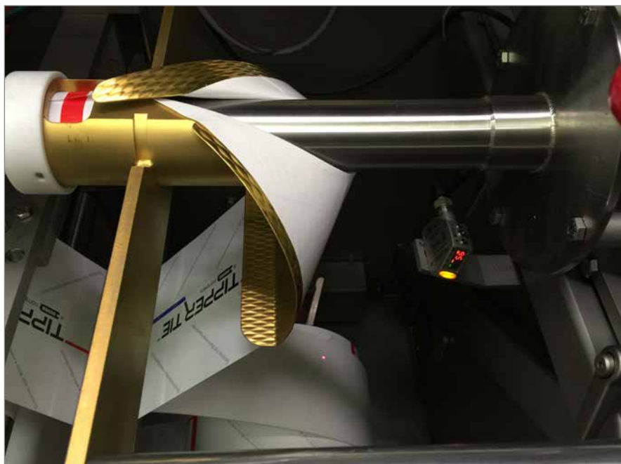
L'épaulement de formage permet un réglage précis du diamètre.
