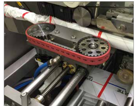
Unité de scellage comportant un réglage de température automatique.
